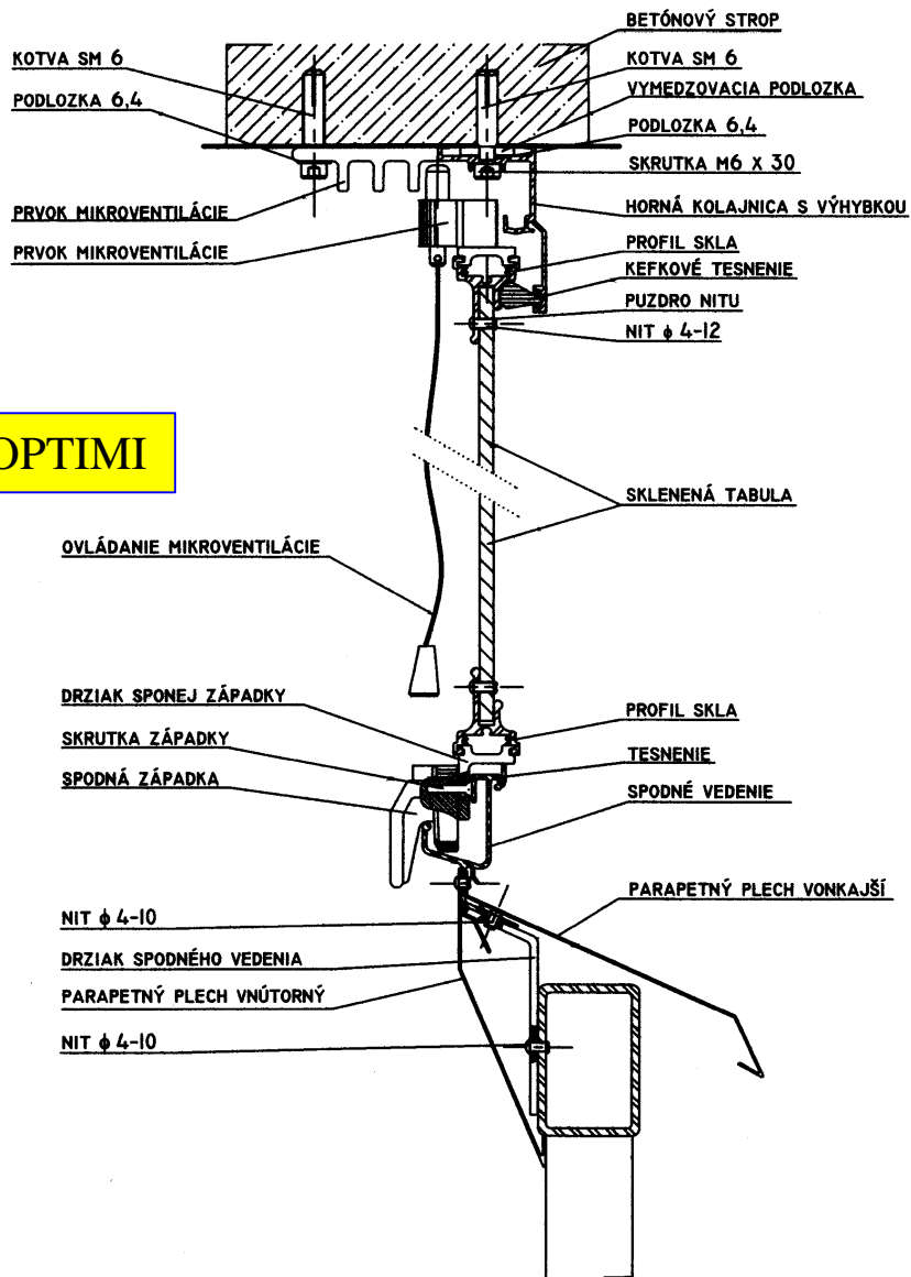
Obr. 2. Priečný rez " B - B " ( detail ovládania uzatvorenia prvého skla a ovládanie mikroventilácie )
