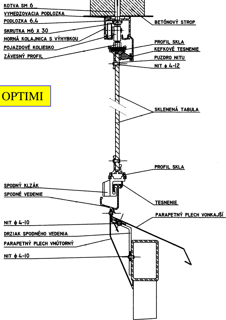
Obr. 1. Priečny rez " A - A " ( detail uloženia a vedenia skla v koľajniciach )
