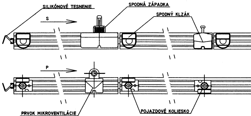
Obr. 5. Detail profilu skiel s vodiacim, tesniacim a uzatváracím prvkom
