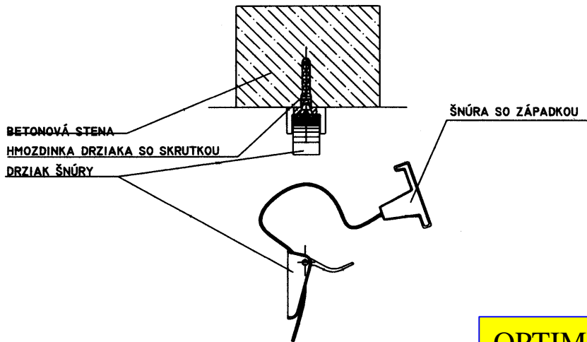
Obr. 4. Detail bočnej aretácie skiel
